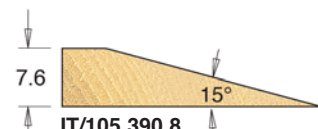
IT/105 390 8 (a = 150°)
