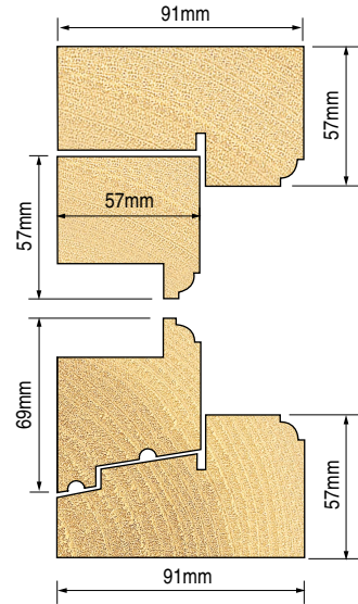
Dimensions
