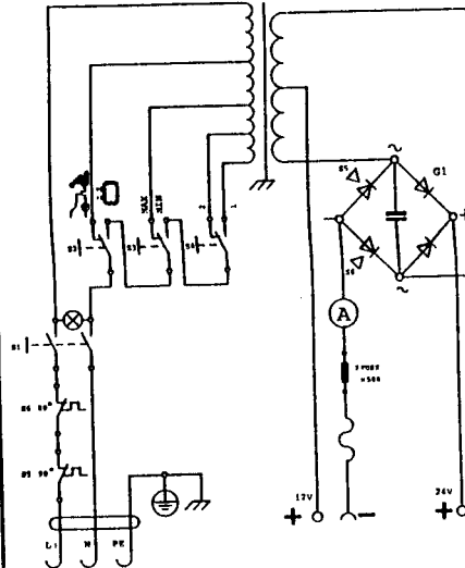
Schema elettrico N. Schéma électrique N. Diagram N. Schaltplan N. Esquema de conexiones N.
