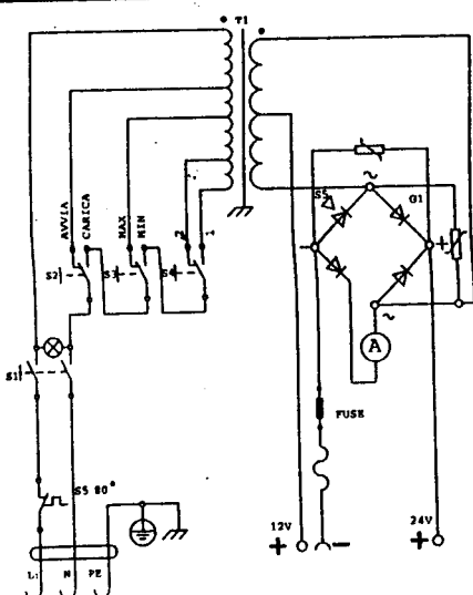
Schema elettrico N. Schéma électrique N. Diagram N. Schaltplan N. Esquema de conexiones N.
